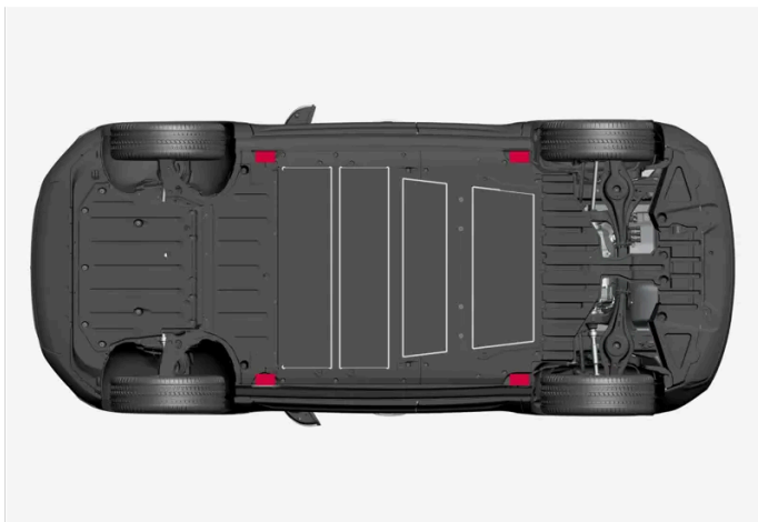
Ansatzpunkte des Fahrzeugs zum Anheben mit einem Wagenheber.
