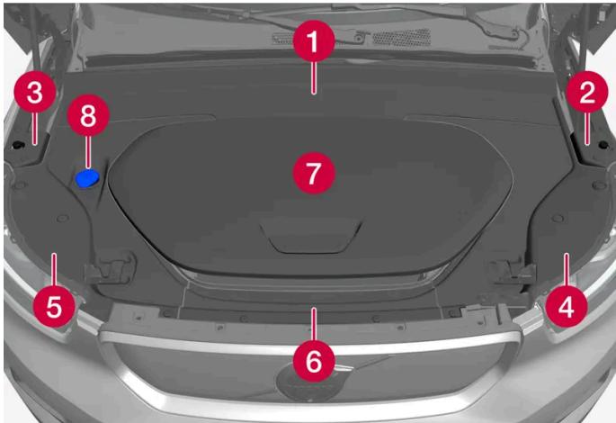
Lage verschiedener Abdeckungen und Teile unter der Frontklappe.
