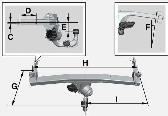
Abmessungen, Befestigungspunkte in mm (Zoll)
