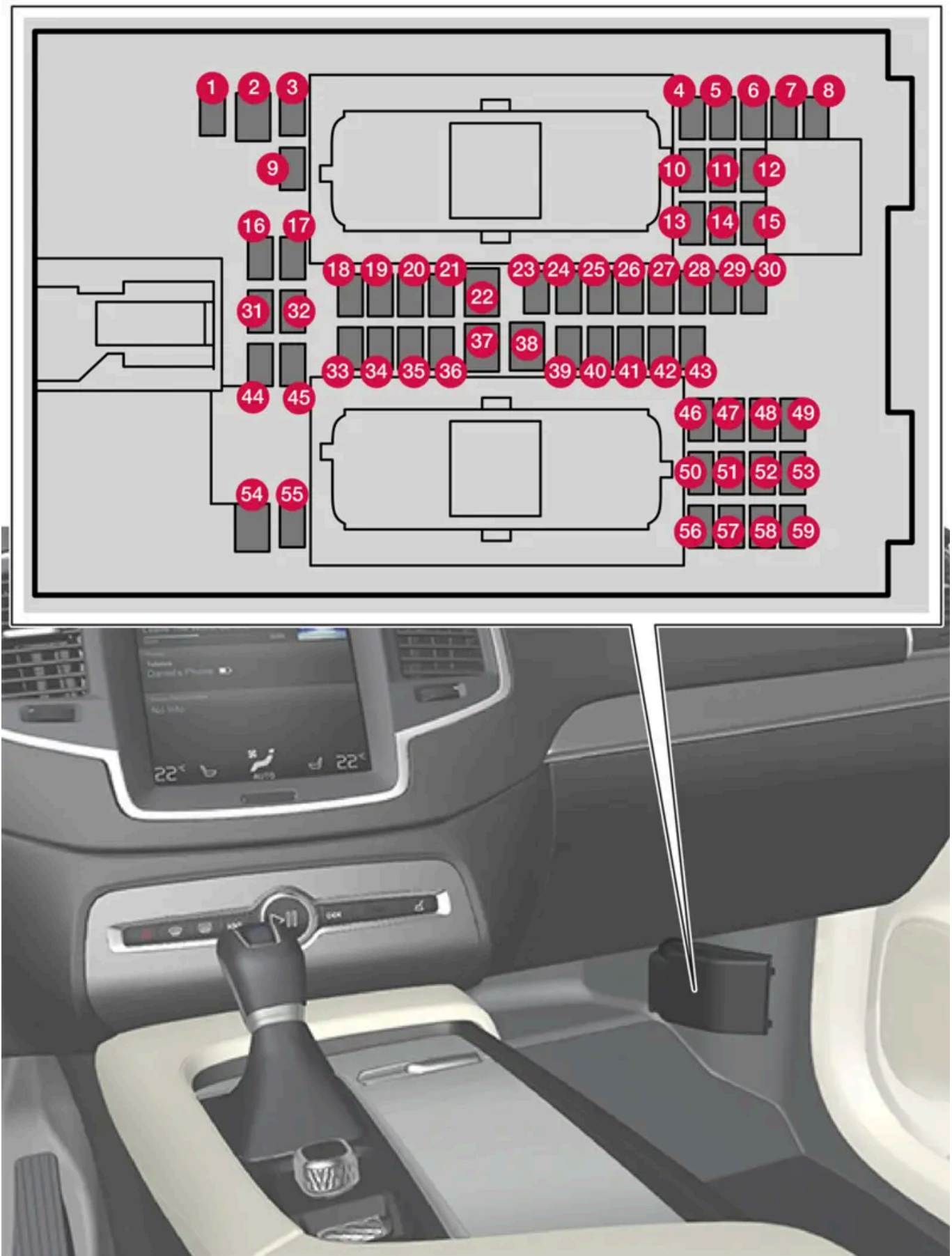
Der Sicherungskasten befindet hinter der Bodenmatte/Seitenverkleidung.
