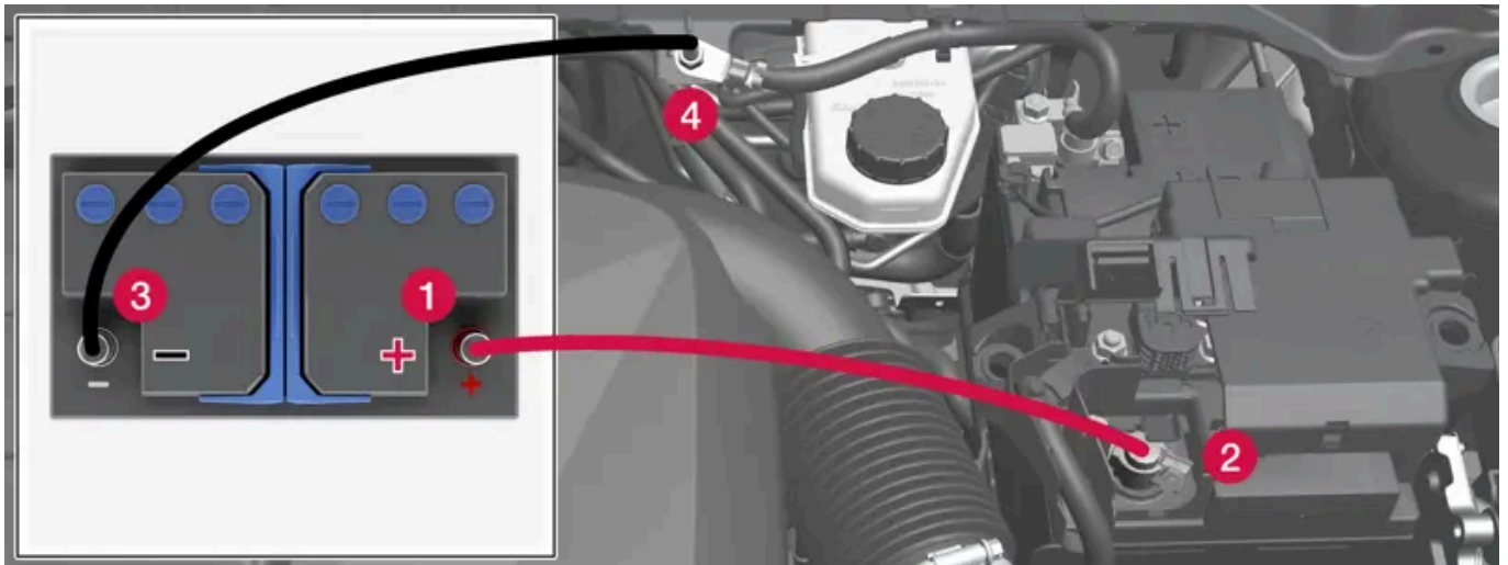
Puntos de fijación de los cables de arranque.
