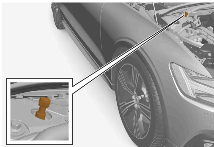
Ubicación del botón giratorio de ajuste de la rueda delantera.
