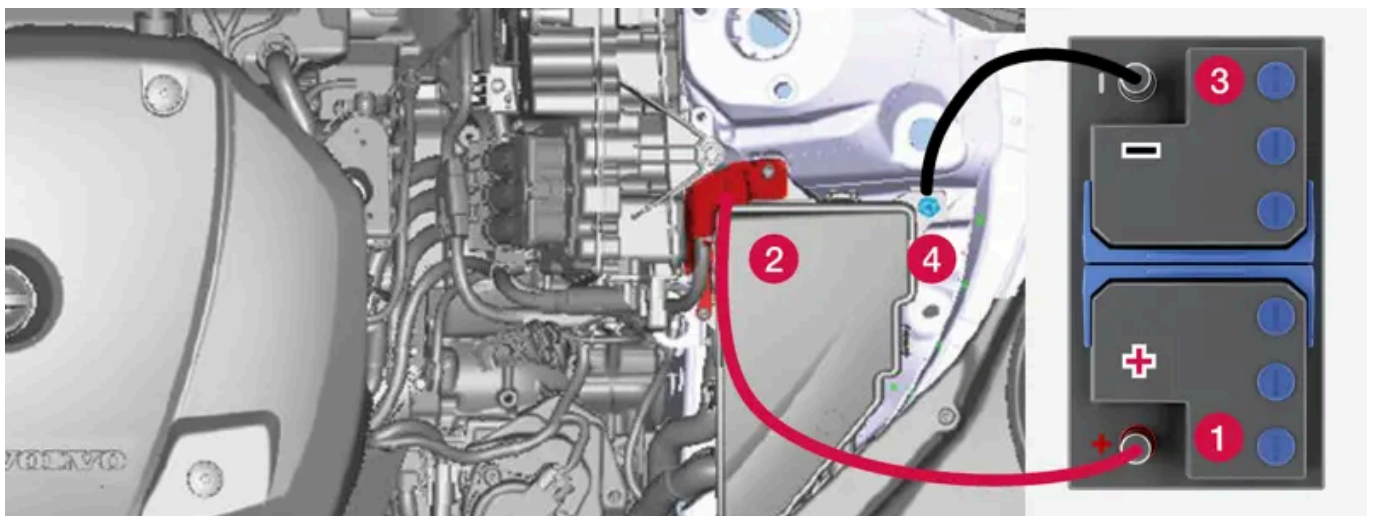
Points de charge pour le démarrage auxiliaire de la voiture. L'aspect du compartiment moteur peut varier selon le modèle de la voiture et le niveau d'équipement.
