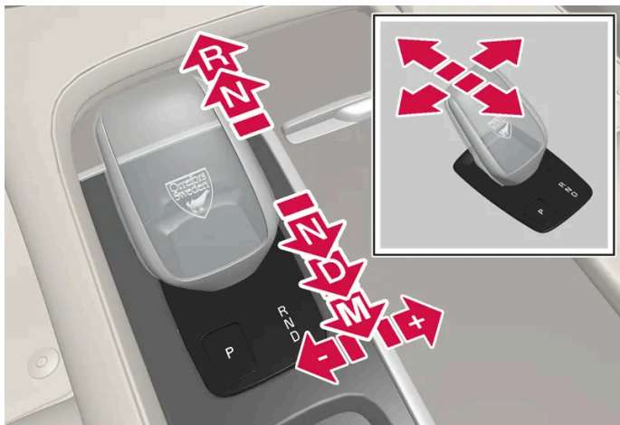
Vue d'ensemble du levier de rapport et des positions de rapport.
