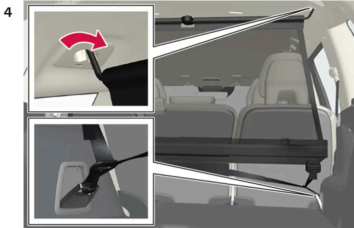
Montage arrière.
