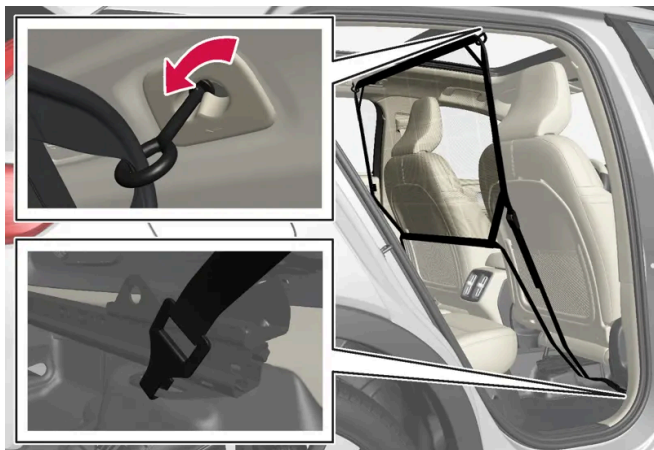
Τοποθέτηση του δικτυού ασφαλείας.
