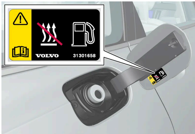
Πινακίδα στο εσωτερικό της θυρίδας ρεζερβουάρ καυσίμων.
