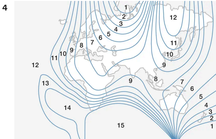
Zone magnetiche.
