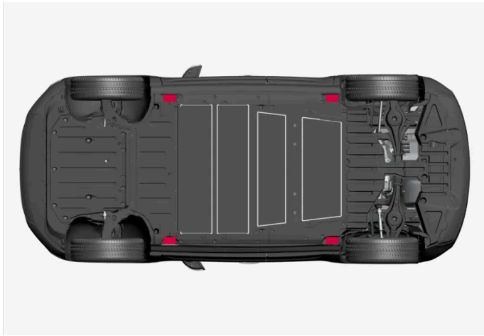
잭을 사용한 차량의 잭업 위치
