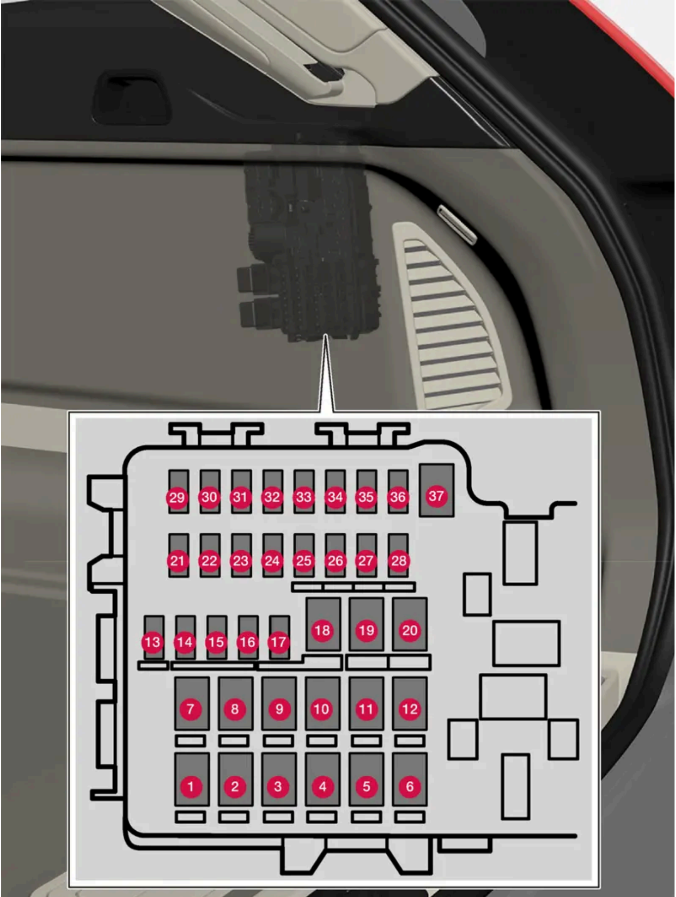
퓨즈박스는 우측의 패널 뒤에 배치되어 있습니다.
