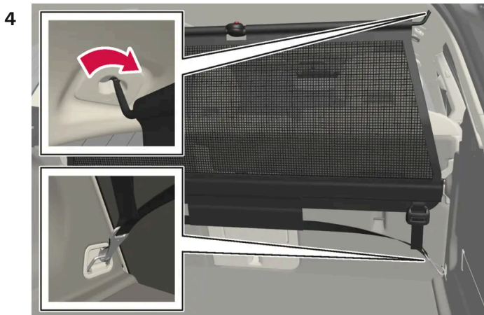
후방에 장착하기. 후방에 장착하기:
