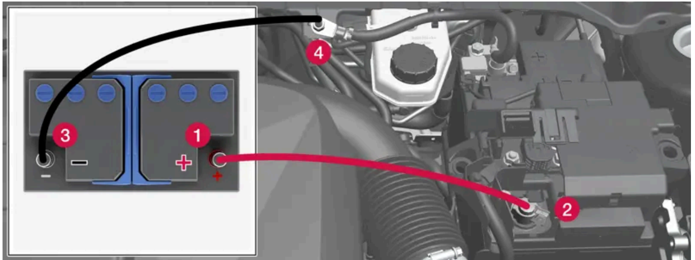
Aansluitpunten voor de startkabels.
