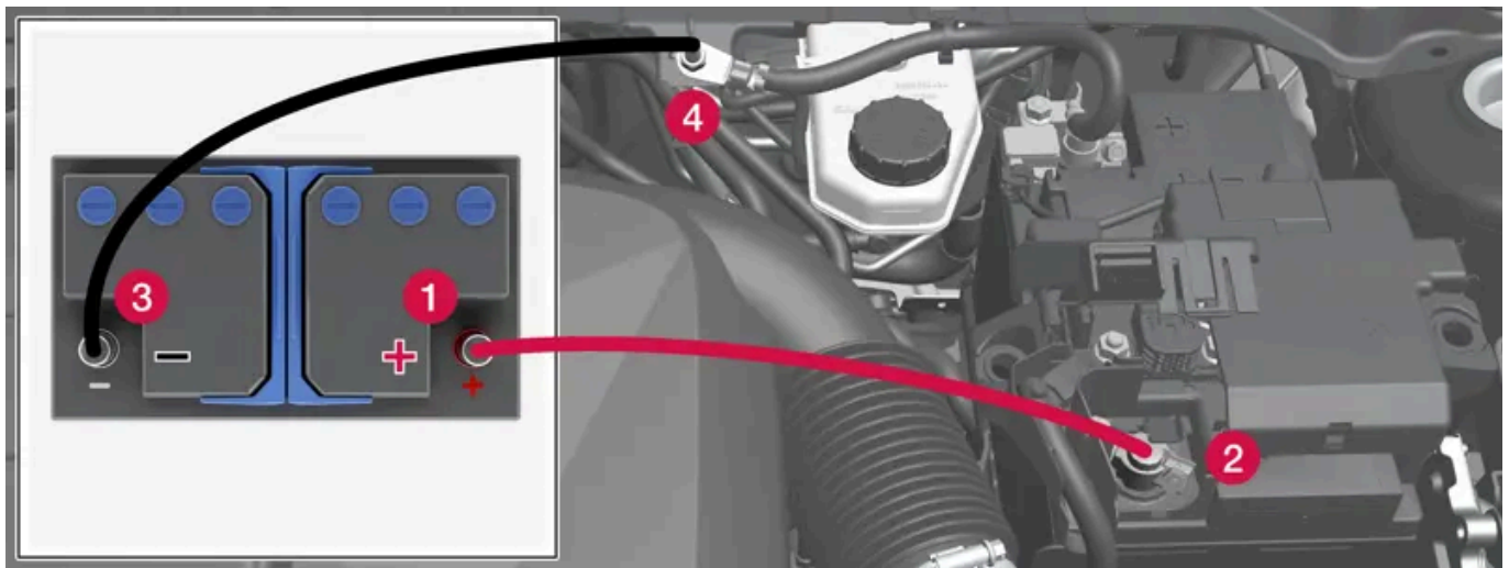
Aansluitpunten voor de startkabels.
