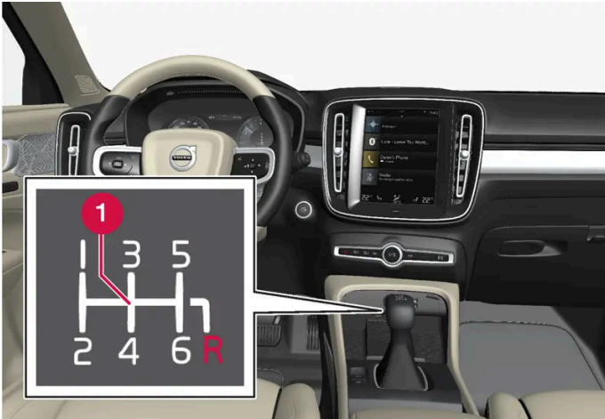
Overzicht schakelhendel en schakelpatroon.
