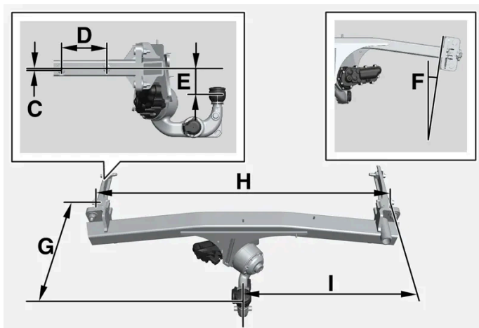
Wymiary, punkty mocowania w mm (calach)
